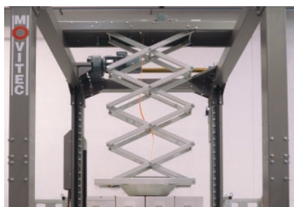
○ Pisón motorizado
